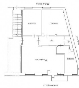
PIANTA PIANO TERRA/RIALZATO HF 3.00 m
