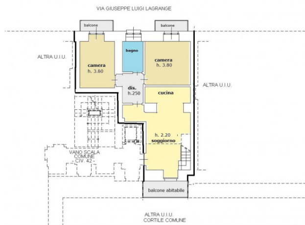
PIANO SOPPALCO su soggiorno
