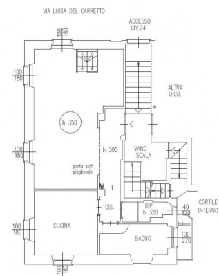
PIANO PRIMO / RIALZATO 1/100 STATO RILEVATO
