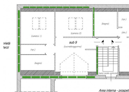
Pianta piano mansardato
