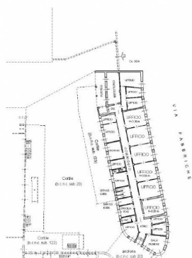
PIANTA PIANO TERRENO H = 3.30 m
