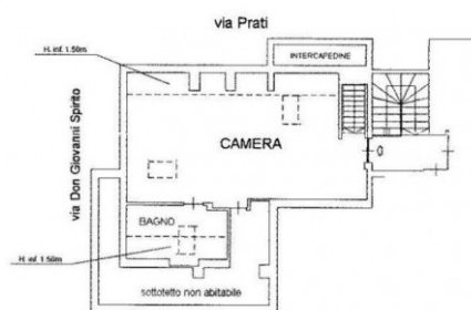
PIANO QUARTO - SOTTOTETTO H. media =2.00 m
