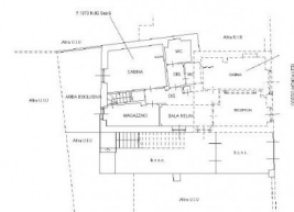
PIANTA PIANO TERRA H = 3.05
