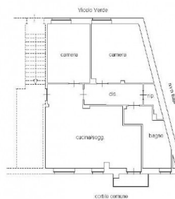
PIANTA PIANO TERRA/RIALZATO H= 3.00 m
