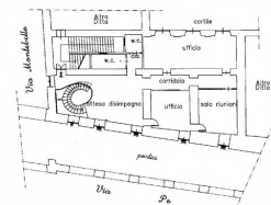
PIANTE PIANO AMMEZZATO altezza mt. 2,50
