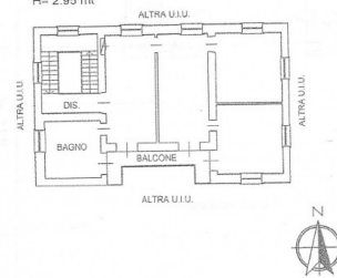
PIANO PRIMO H= 2.95 mt
