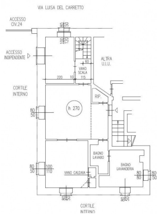
PIANO TERRA / SEMINTERRATO 1/100 STATO RILEVATO
