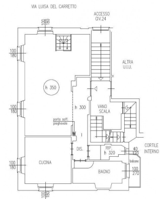
PIANO PRIMO / RIALZATO 1/100 STATO RILEVATO
