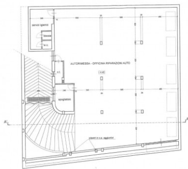
Piano interrato (nessuna variazione in progetto)
